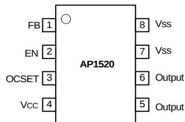
SO-8
