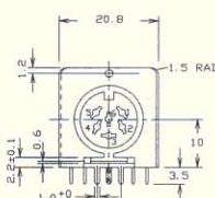
D6 6 Pin 240° right angle PCB mounting DIN socket.
