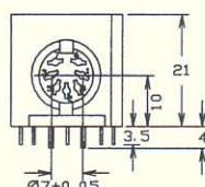
D7 7 Pin right angle PCB mounting DIN socket.
