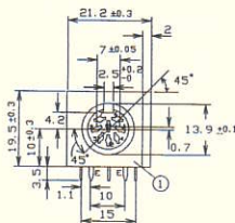
D8 8 Pin right angle PCB mounting DIN socket.
