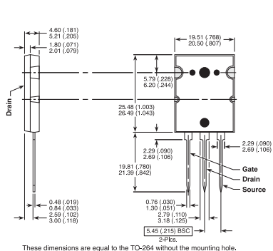
264 MAX ™
