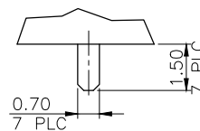
DETAIL D 2:1
