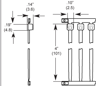
AT2000 Cable Ties
