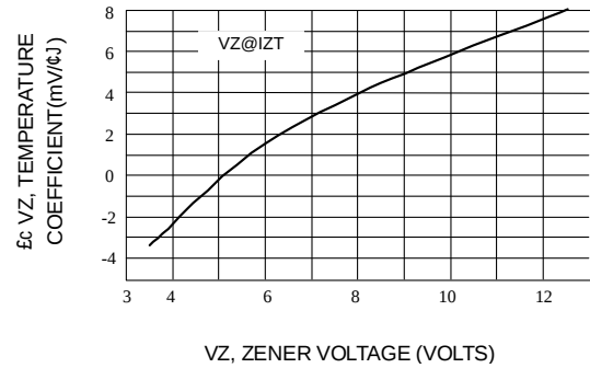
Fig. 2-ZENER VOLTAGE-TO 12 VOLTS
