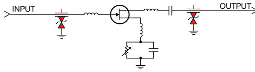
Fig. 4 – GaAs FET Protection
