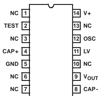
ICL7662 (PDIP) TOP VIEW
