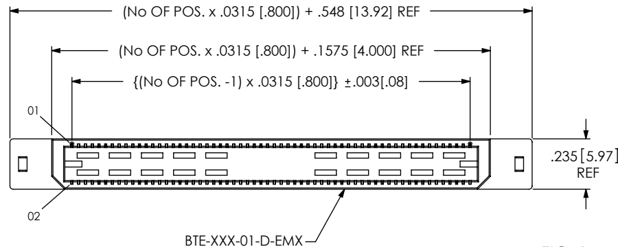
FIG. 1 BTE-060-01-X-D-EM2 SHOWN
