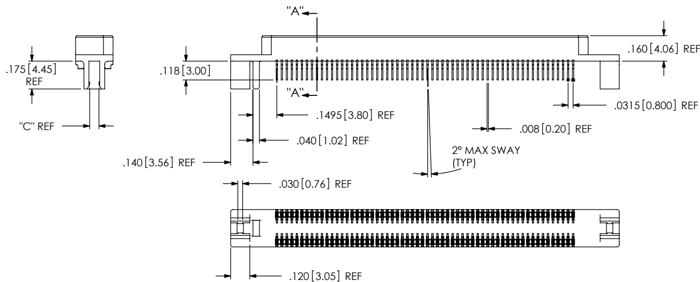
FIG. 1 BTE-060-01-X-D-EM2 SHOWN
