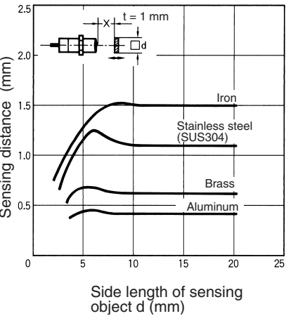
E2E-X1R5E/V E2E-X1R5Y
