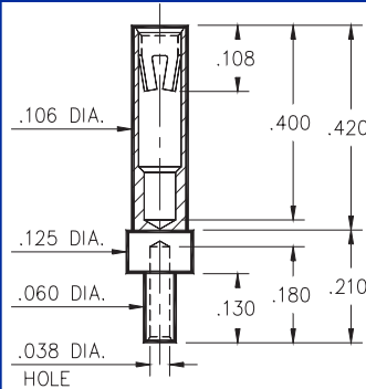
8730-0-19-XX-23-XX-10-0 Wire Termination
