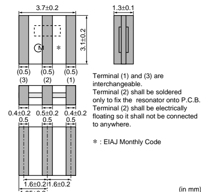
CSACV_X_Q 14.70-70.00MHz
