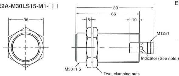
E2A-M30LS15-M1-□□
