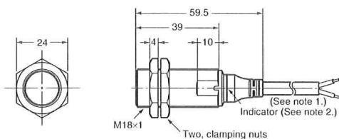
E2A-M18KS08-WP-□□
