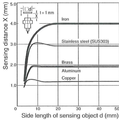
E2A-S08□N04/M08□N04
