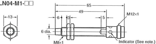
E2A-S08LN04-M1-□□ E2A-M08LN04-M1-□□
