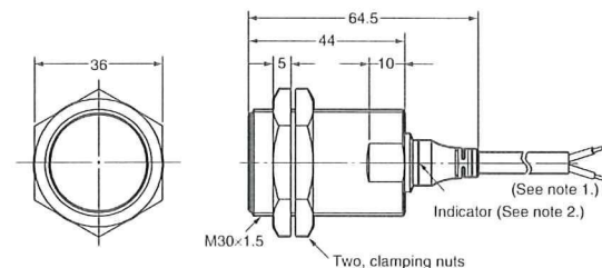
E2A-M30KS15-WP-□□
