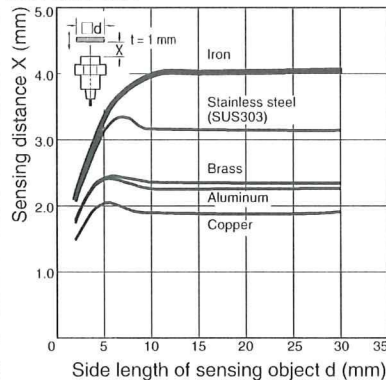
E2A-M12 S04
