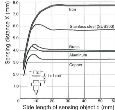
E2A-M18 S08
