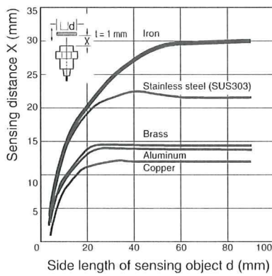
E2A-M30LN30
