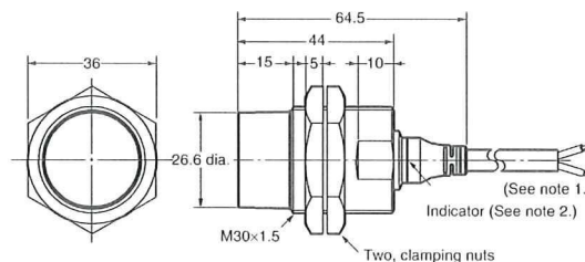
E2A-M30KN20-WP-□□
