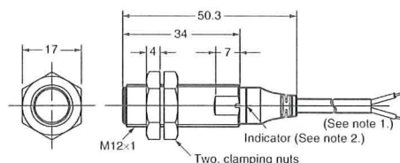
E2A-M12KS04-WP-□□
