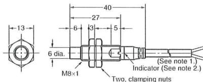
E2A-S08KN04-WP-□□
