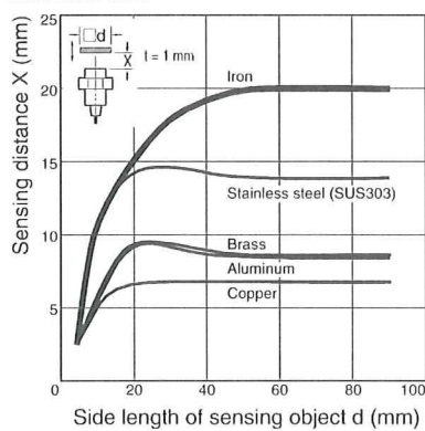
E2A-M30KN20
