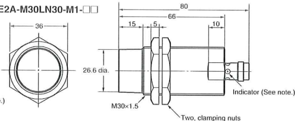
E2A-M30LN30-M1-□□
