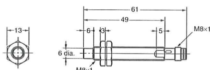
E2A-S08LN04-M5-□□
