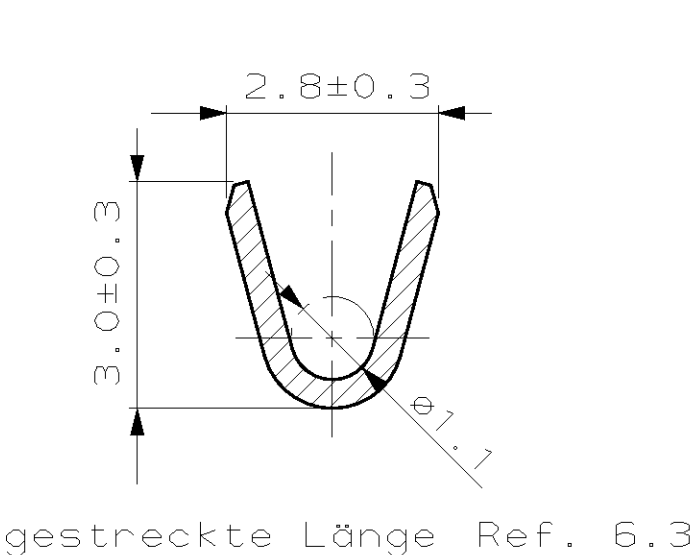
Schnitt C-C
