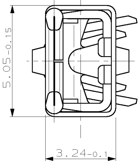
ANSICHT X
