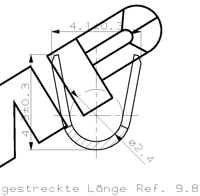
Schnitt B-B
