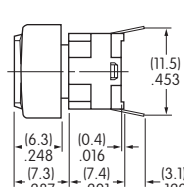
Extended Actuator
