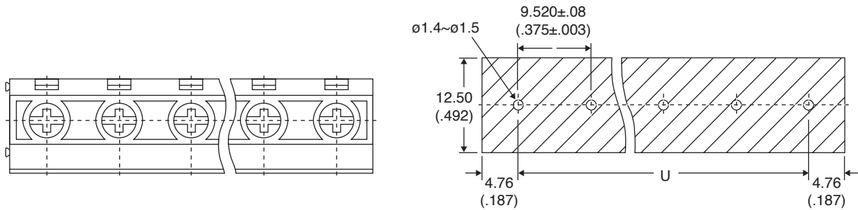
P.C.B. LAYOUT (REF)
