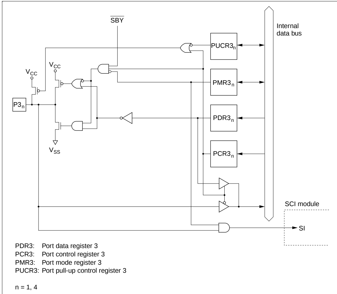
Figure C.3 (d) Port 3 Block Diagram (Pins P3_4 and P3_l )
