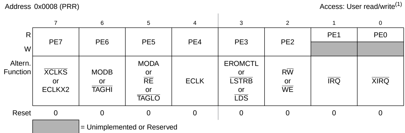
Figure 19-9. Port E Data Register (PORTE)
