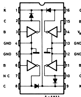
ULN2069B ULN2071B
