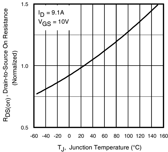
Q1 - Control FET
