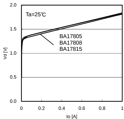
Fig.19 出力電流－最小出力電圧差
