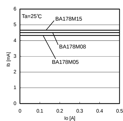
Fig.12 出力電流－バイアス電流
