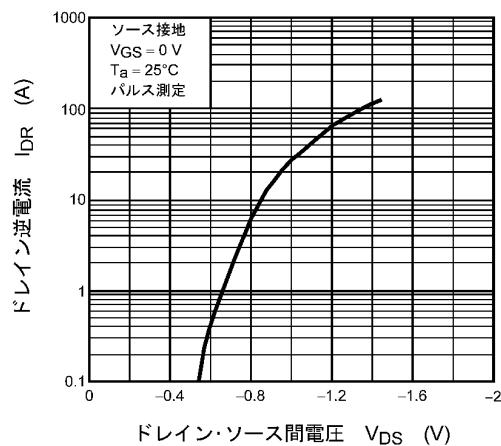
図 8.8 I_{DR} - V_{DS}
