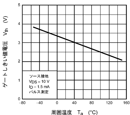
図 8.11 V_{th} - T_a
