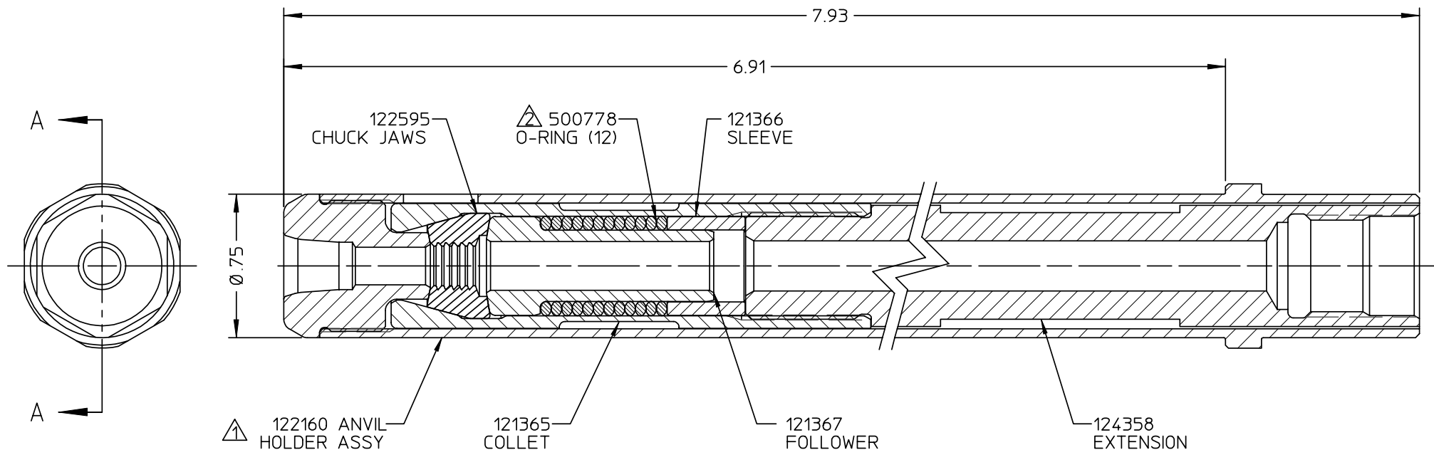
SECTION A-A
