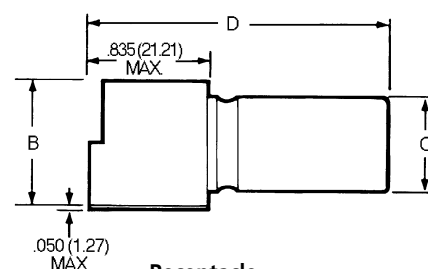
Receptacle
