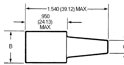
Receptacle P/N 120-1833-000
