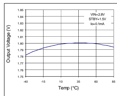
Fig 11. VOUT - Temp
