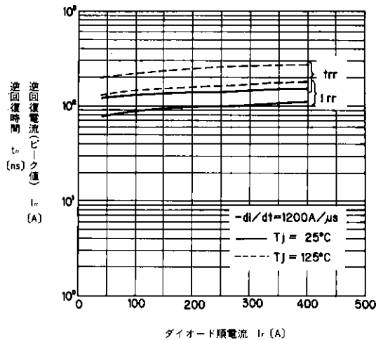
ダイオード順電流 I_r (A) t_{rr} , I_{rr} - I_r 特性 T_{rr} , I_{rr} - I_r
