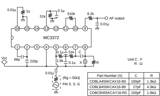
MC3372
