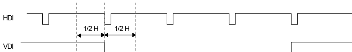
Fig. 115 HDI VDI Input Timing
