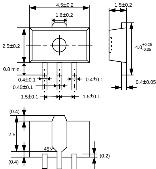
(3) SOT-89-3
