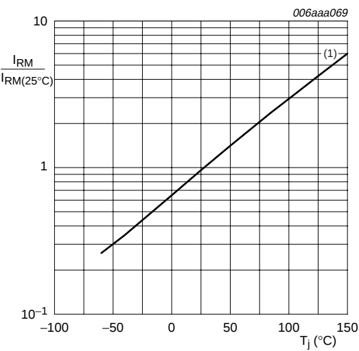
(1) PESD3V3L2BT, PESD5V0L2BT PESD12VL2BT, PESD15VL2BT and PESD24VL2BT: I_{RM} < 20\text{ nA} ; T_j = 150\text{ }^{\circ}C
