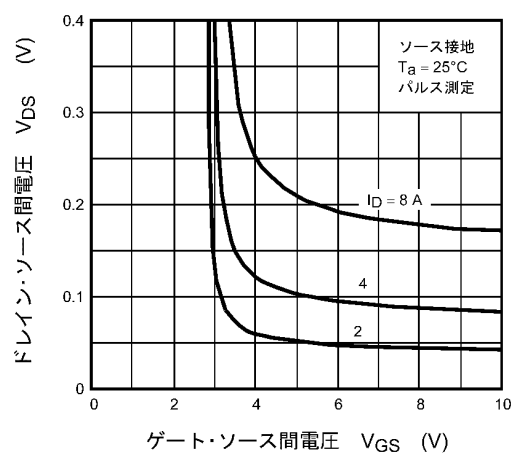
図 8.4 V_{DS} - V_{GS}
