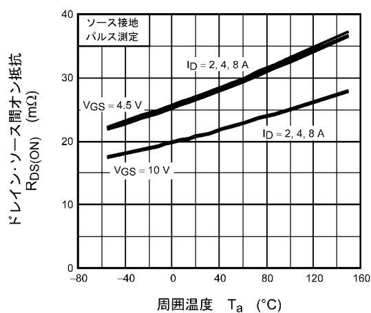
図 8.6 R_{DS(ON)} - T_a
