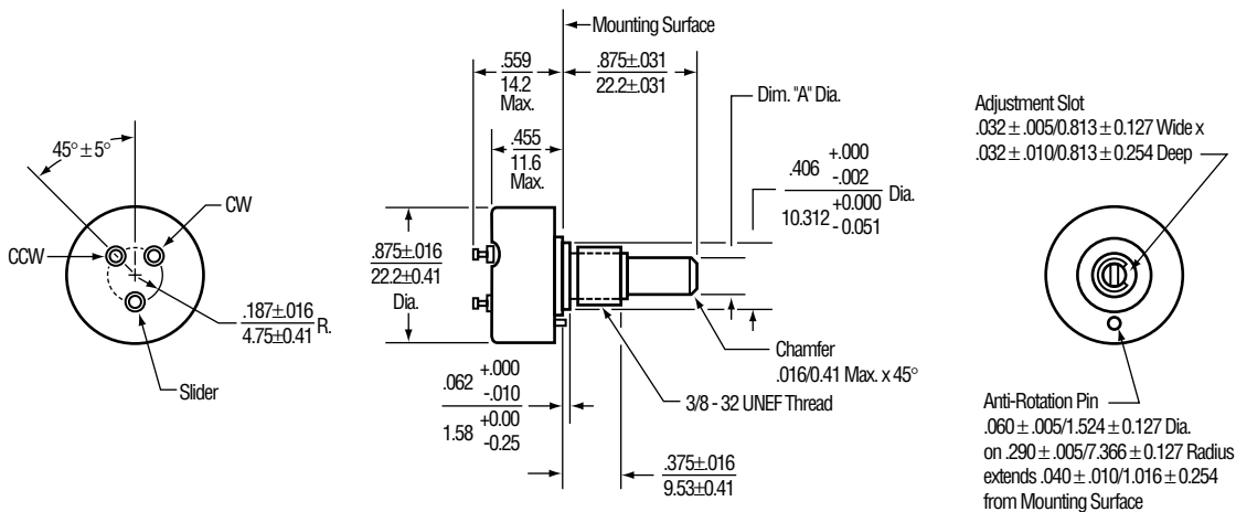
Model 6186 & 6187
