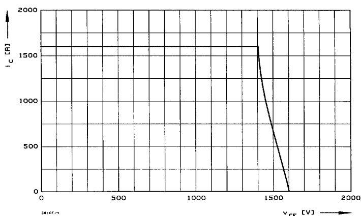
4 Rückwärts-Arbeitsbereich RBSOA. Reverse biased safe operating area. t_{vj} = 125^\circ\text{C} , V_{LF} = V_{LR} = 15\text{ V} , R_{GF} = 5,6\ \Omega , R_{GR} = 2,4\ \Omega
