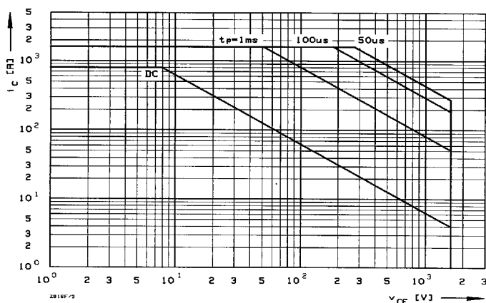
3 Vorwärts-Arbeitsbereich FBSOA (Einzelimpuls, nicht periodisch). Forward biased safe operating area (single pulse, non repetitive). t_{vj} = 150^\circ\text{C} , t_C = 25^\circ\text{C}
