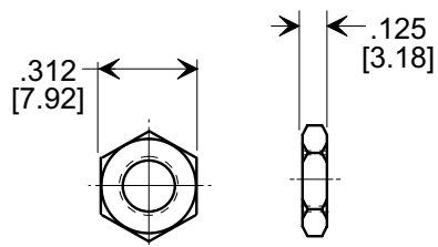
HEX NUT
