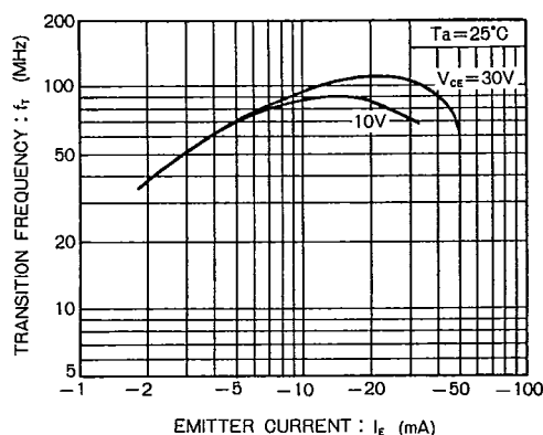
Fig. 10 利得帯域幅積—エミッタ電流特性
