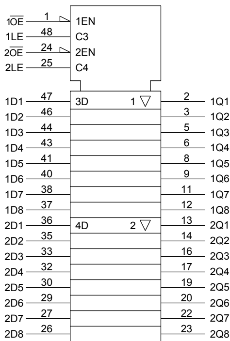
論理図
