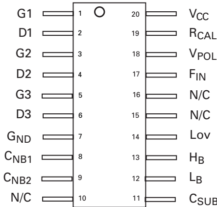
QSOP20
