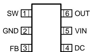
TSOT23-6 (D)
