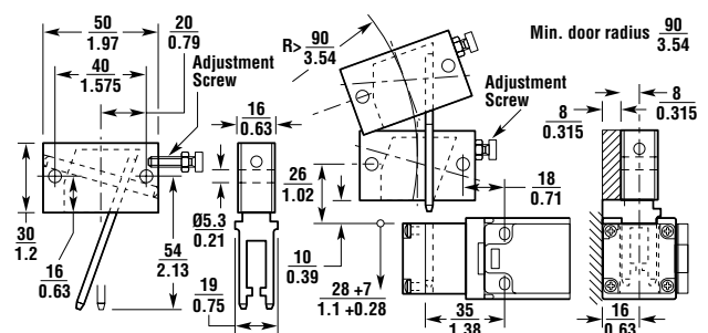
Flexible 2 Actuator
