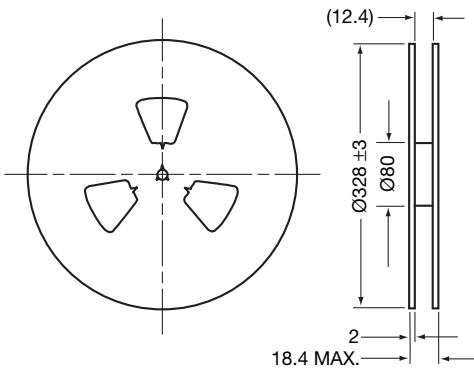
REEL DIMENSIONS
