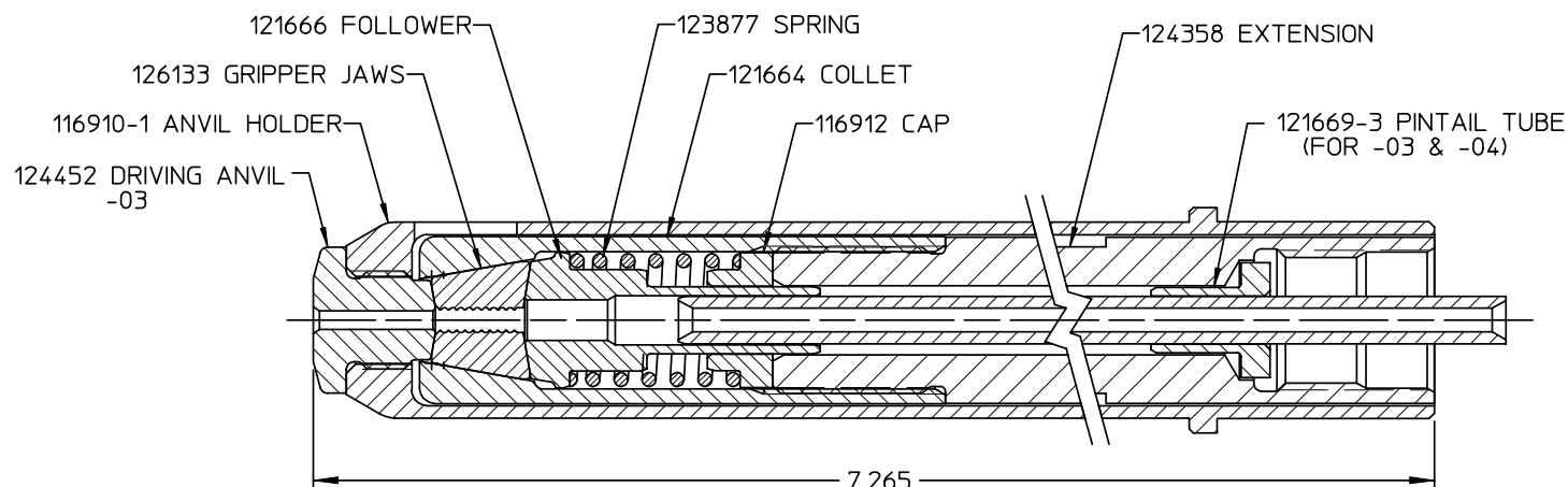
SECTION A-A
