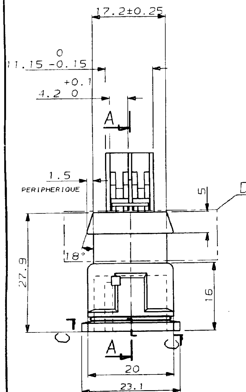
DETAIL D: PARTIE SUPERIEURE PORTE-MODULE
