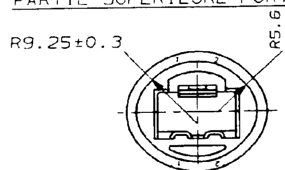
DETAIL D: PARTIE SUPERIEURE PORTE-MODULE
