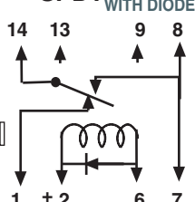
SPDT
