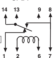
SPDT
