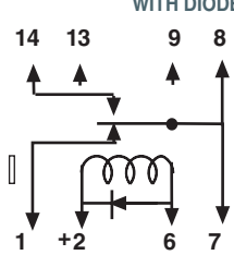
SPDT
