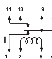
SPDT
