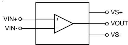
TSOT-23-5 RT9148
