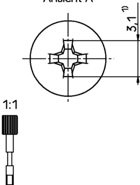
Ansicht A
