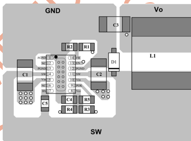
Top Layer
