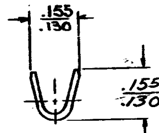
SECT A-A
