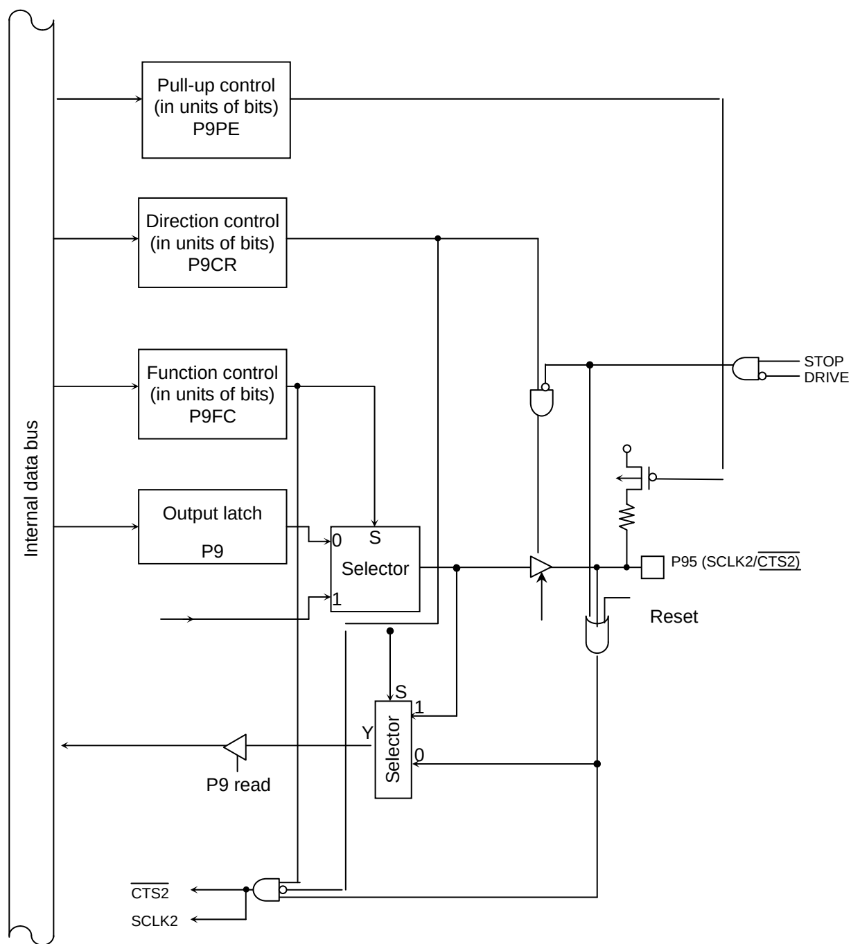
Fig. 7-29 Port 9 (P95)
