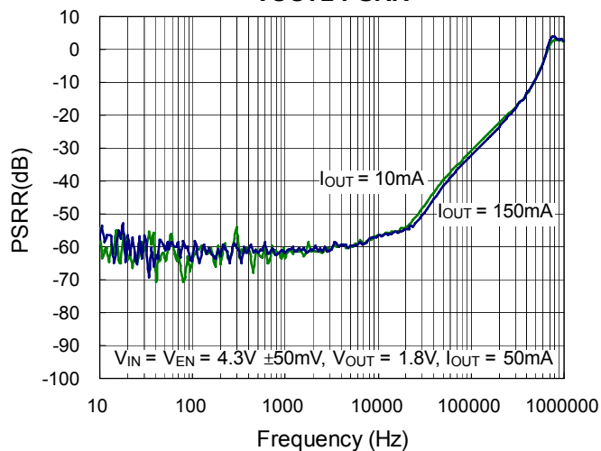
VOUT1 PSRR
