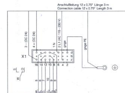
Abb. 4.6 Anschlußbelegung Führungsrahmen SK 3357 100, SK 3358 100 für Einschublüfter Vario
